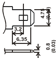
F1 (FASTON TAB NO. 187)
