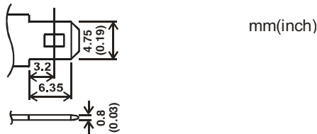
F1 (FASTON TAB NO. 187)
